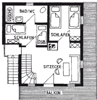
Obergeschoss
